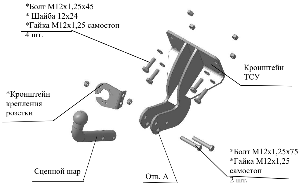
Рис.1 Тягово-сцепное устройство 9311.
