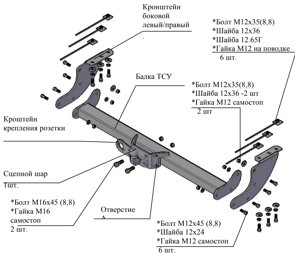
Рис.1 Тягово-сцепное устройство 6050 .
