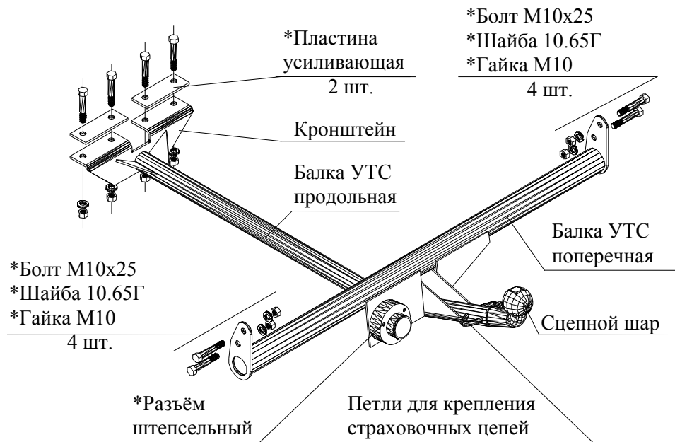
Рис.1 Устройство тягово-сцепное УТС 2106
