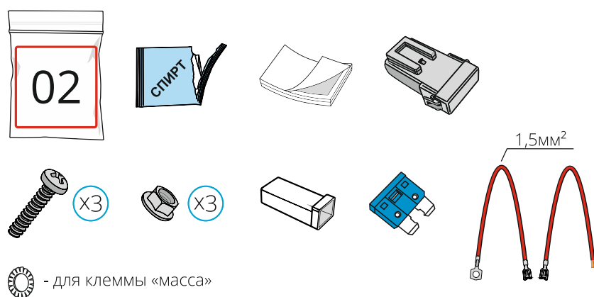
Монтажный комплект
