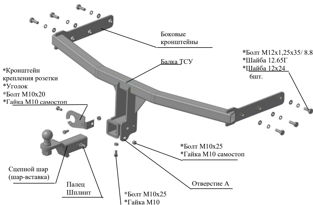
Рис.1 Тягово-сцепное устройство 8125
