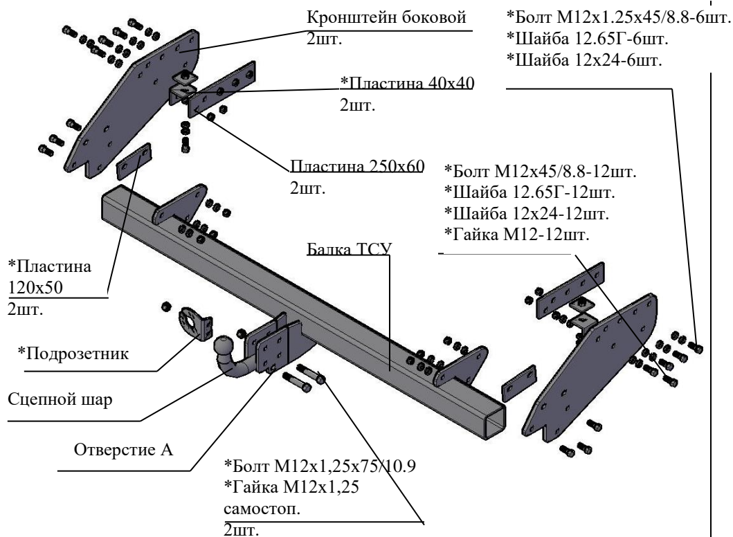
Рис.1 Тягово-сцепное устройство 7112, 7112.Ц
