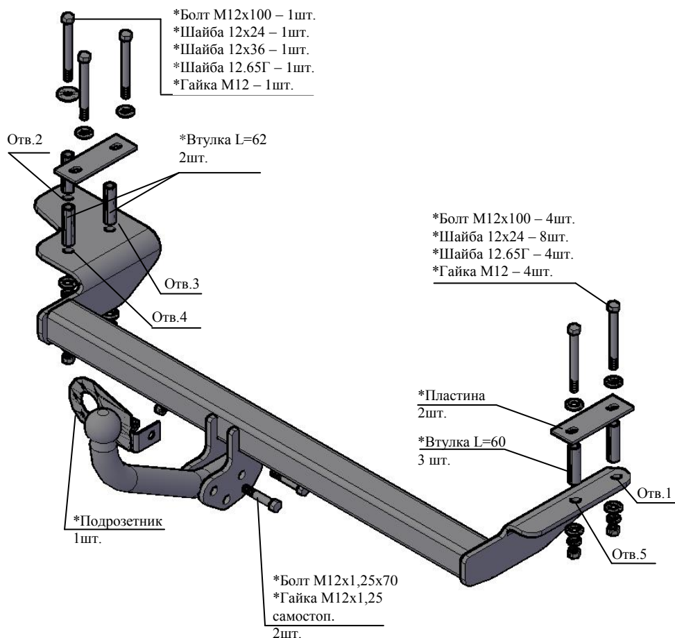
Рис.1 Тягово-сцепное устройство 9410
